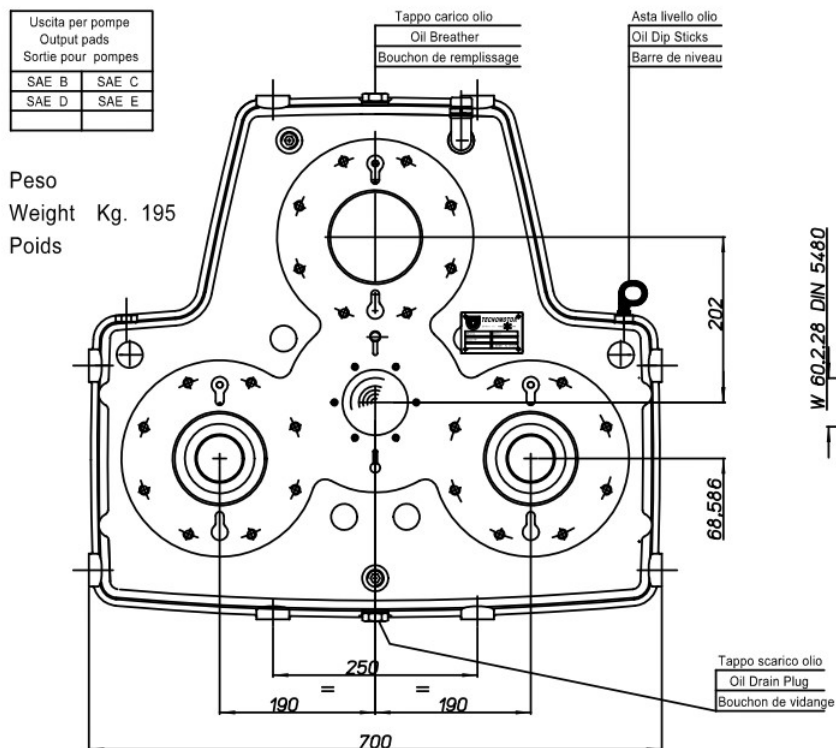
TMP 350 Dimensioni
