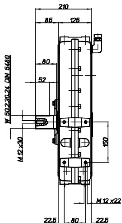
TMP 340 Dimensions
