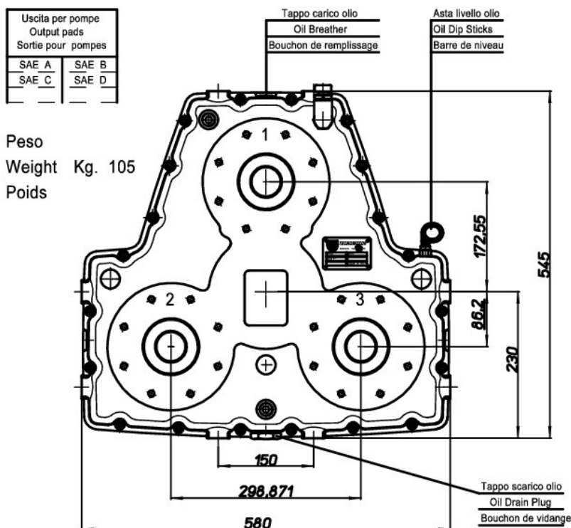
TMP 340 Dimensioni
